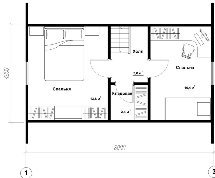
План 2 этажа
