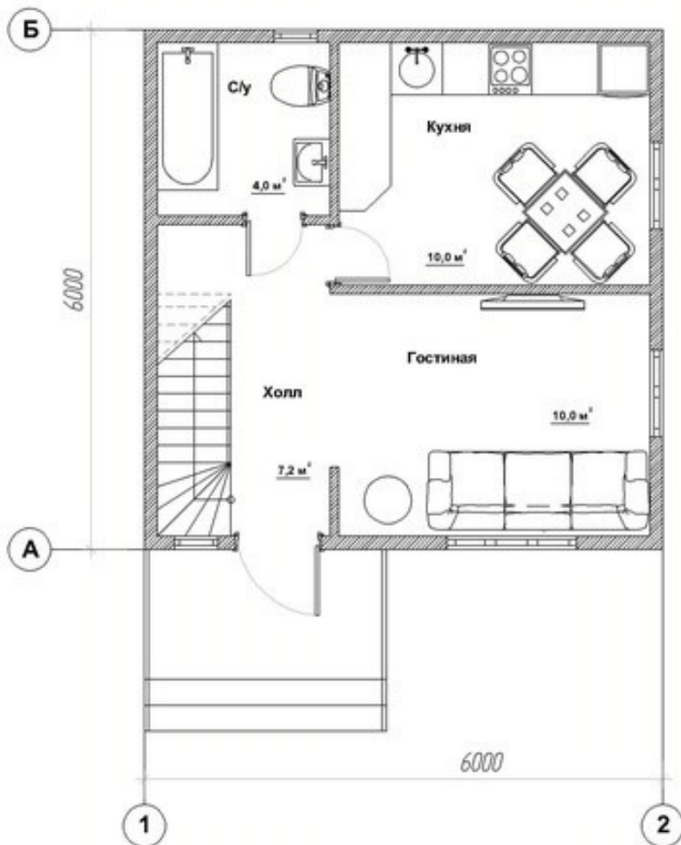
План 1 этажа
