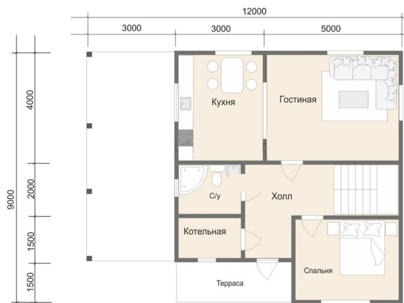
План 1 этажа
