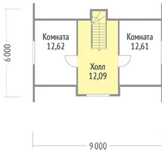
Мансарда
