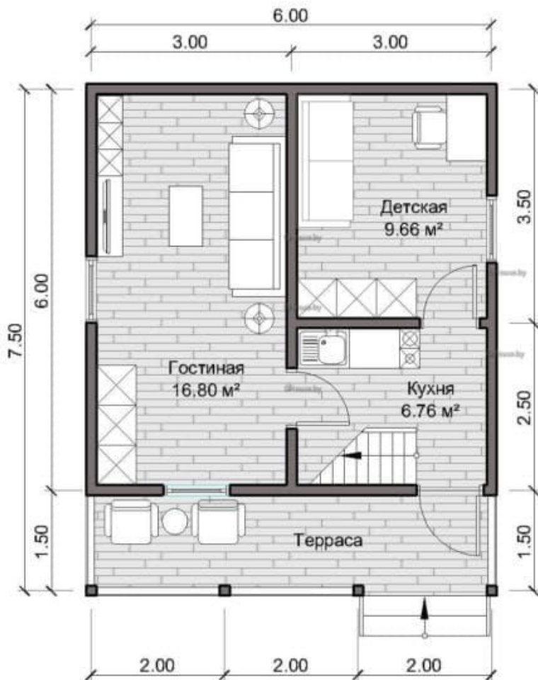
1 этаж
