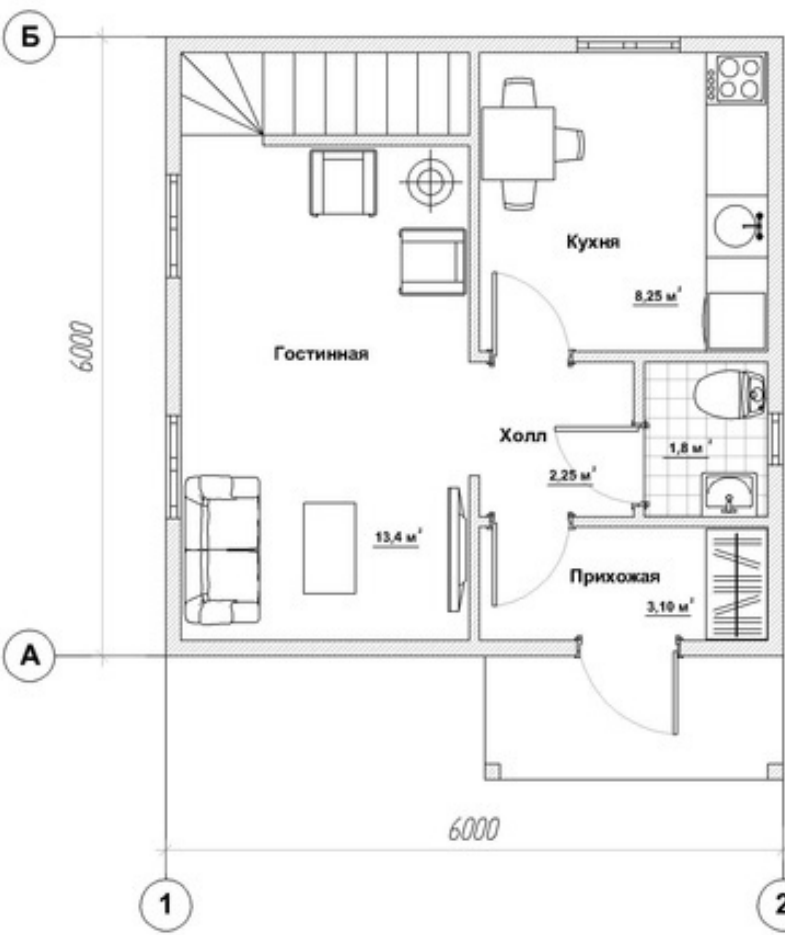
План 1 этажа
