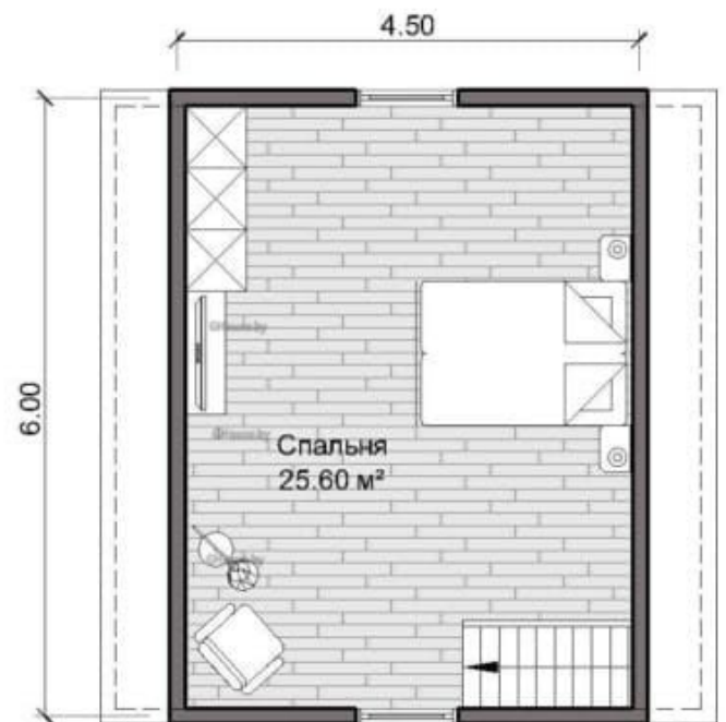
2 этаж
