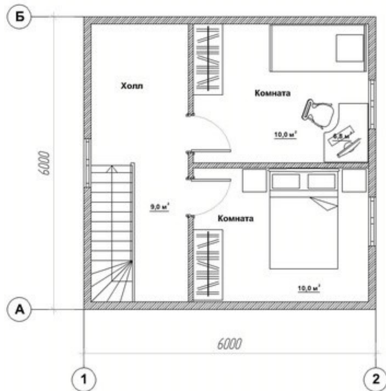
План 2 этажа
